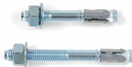
Fixanker gerissener Beton Art.-Nr. 5928 208 015
