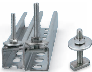
VARIFIX® Hammerkopfbefestiger Rohrinstallation Art.-Nr. 08621 000..
